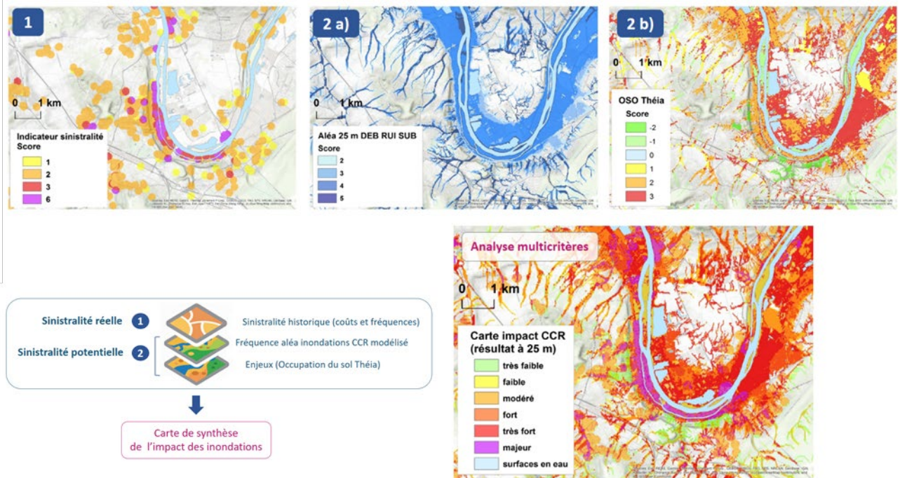
Figure 11 - Superposition des indicateurs et carte de synthèse de l'impact des inondations
